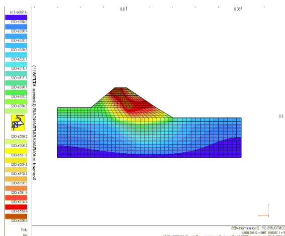
3. Modélisation par éléments finis du profil de digue type. Instabilité du parement « eau » lors d'une vidange rapide préliminaires
